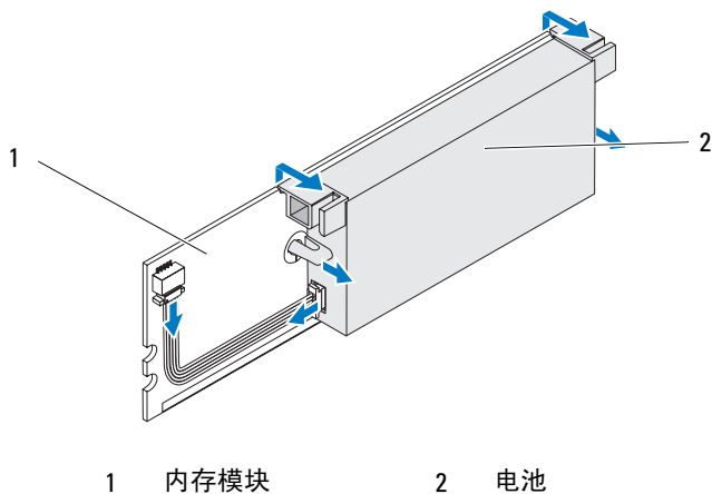
图 2. 卸下 BBU
